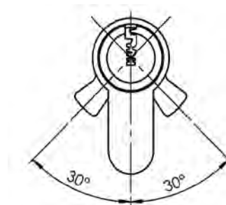
Zulässige Schlüsselabzugsstellung
