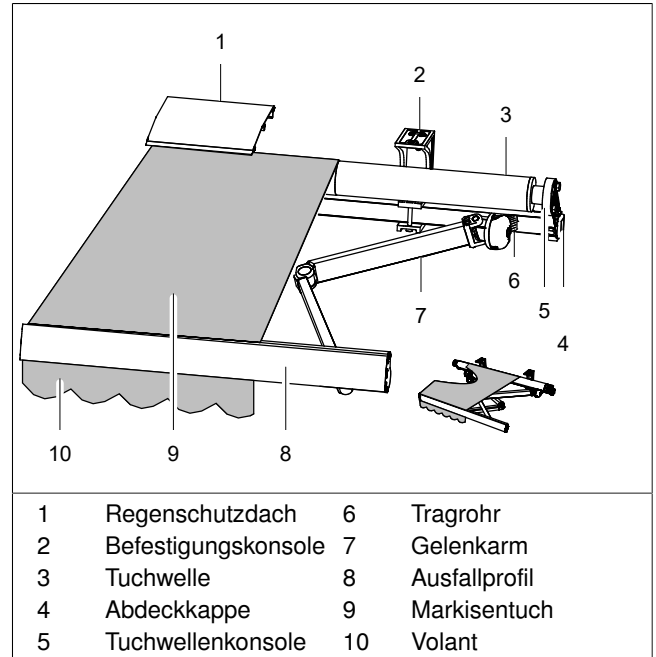
Abb. 1: Teileübersicht Gelenkarm-Markise Typ 530/530 LB
